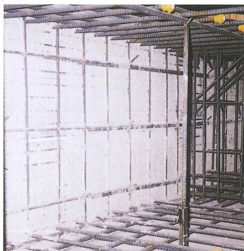
耐圧盤止枠
