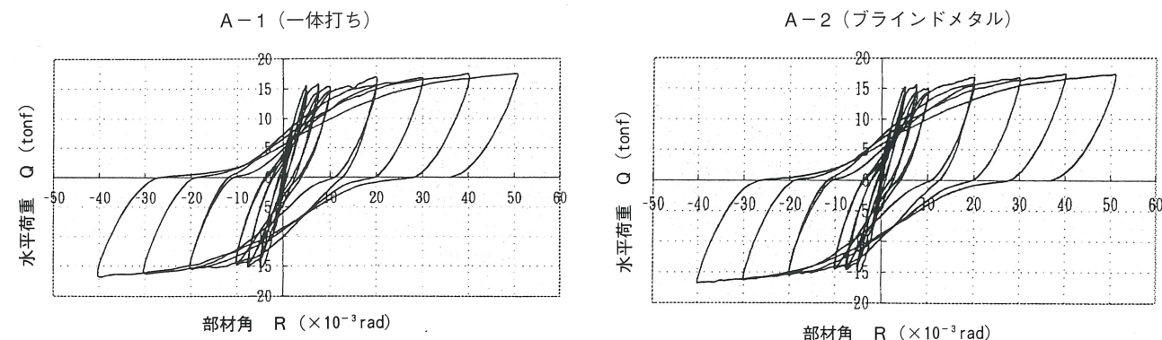
水平荷重 (Q) ・ 変形部材角 (R) の関係表
